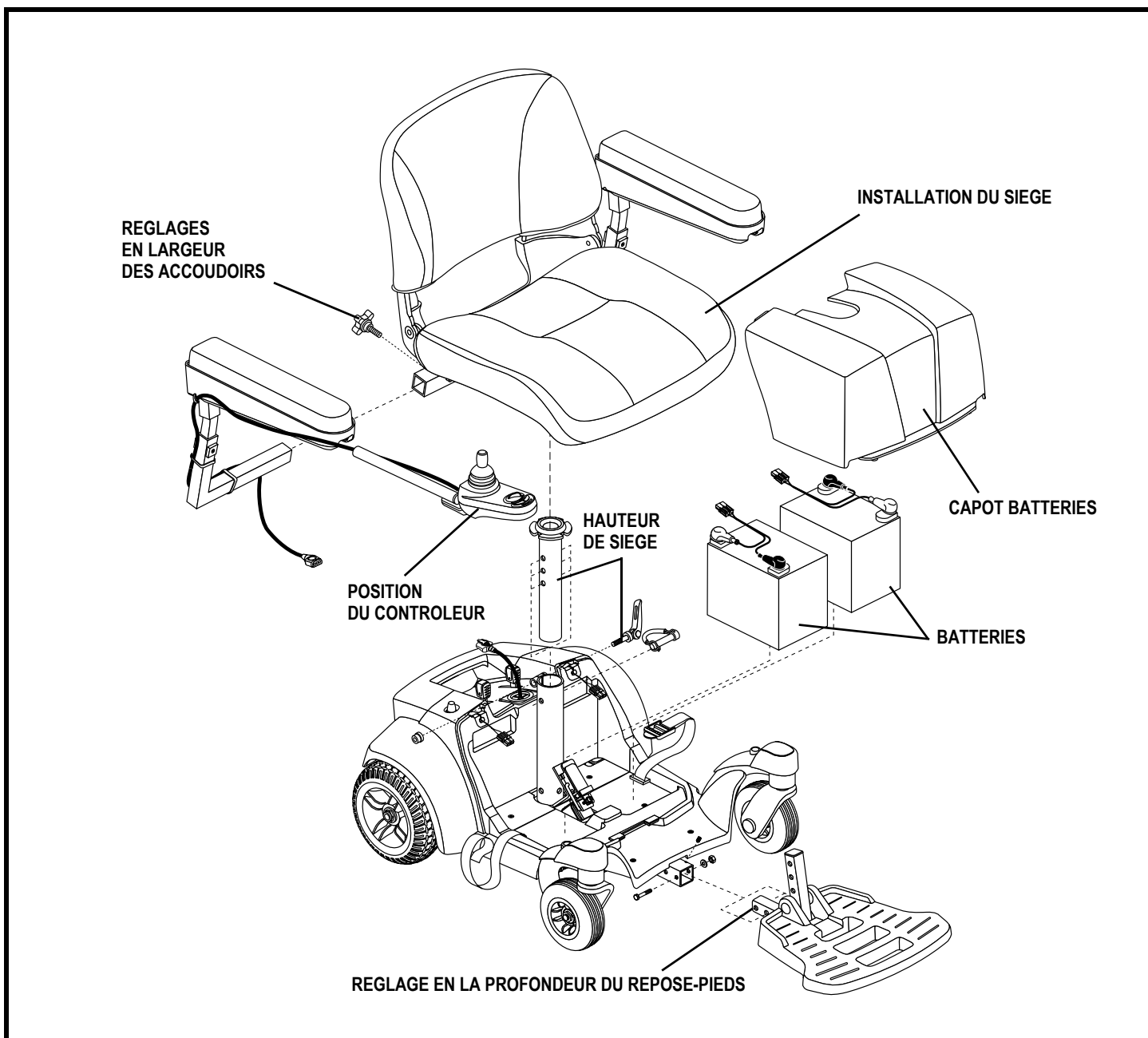
Figure 8. L'assemblage du Select Traveller
