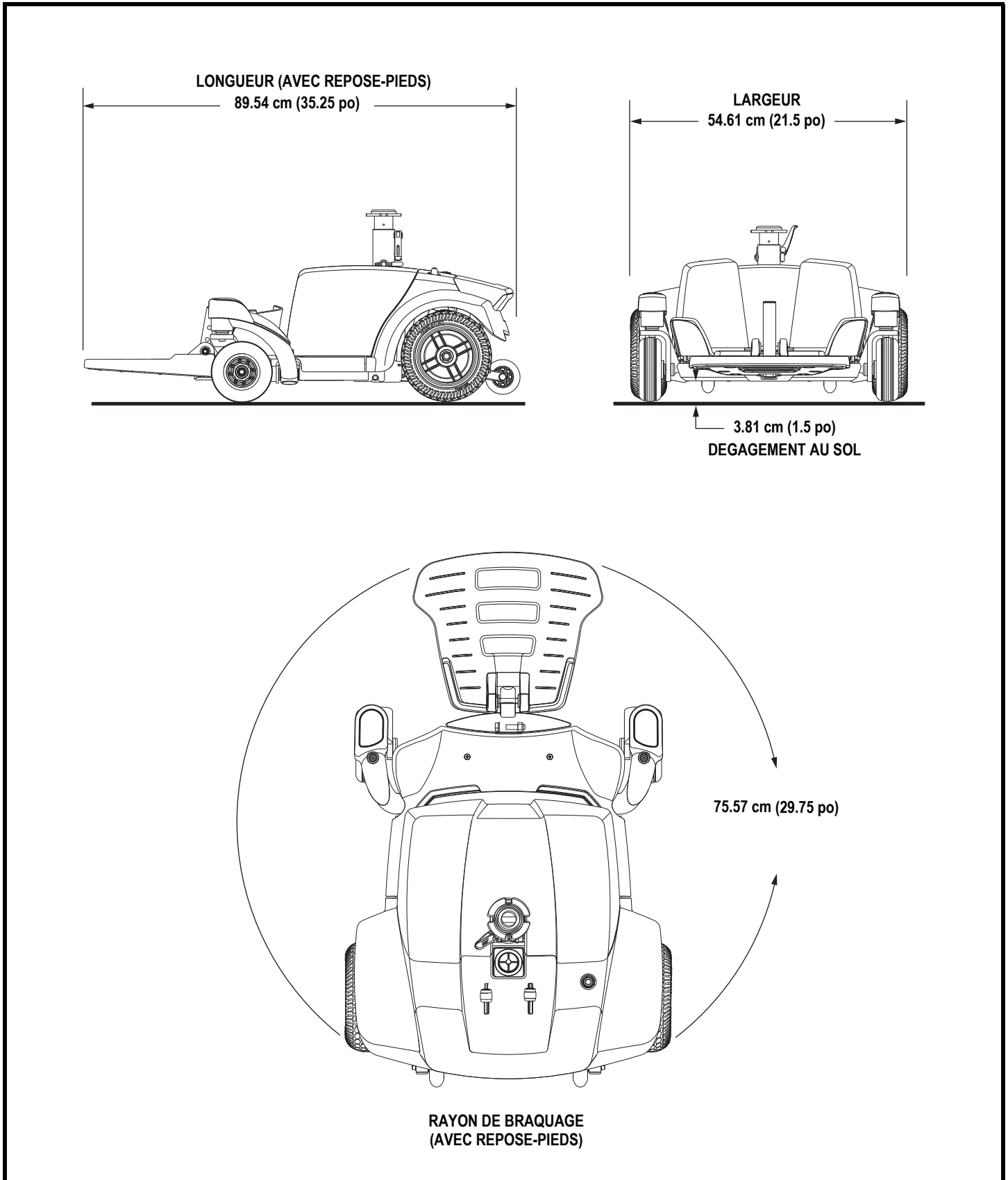
Figure 19. Dimensions et dégagement au sol Select Traveller
