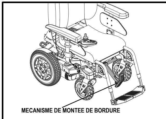
Figure 7. Lightning avec montée de bordure
