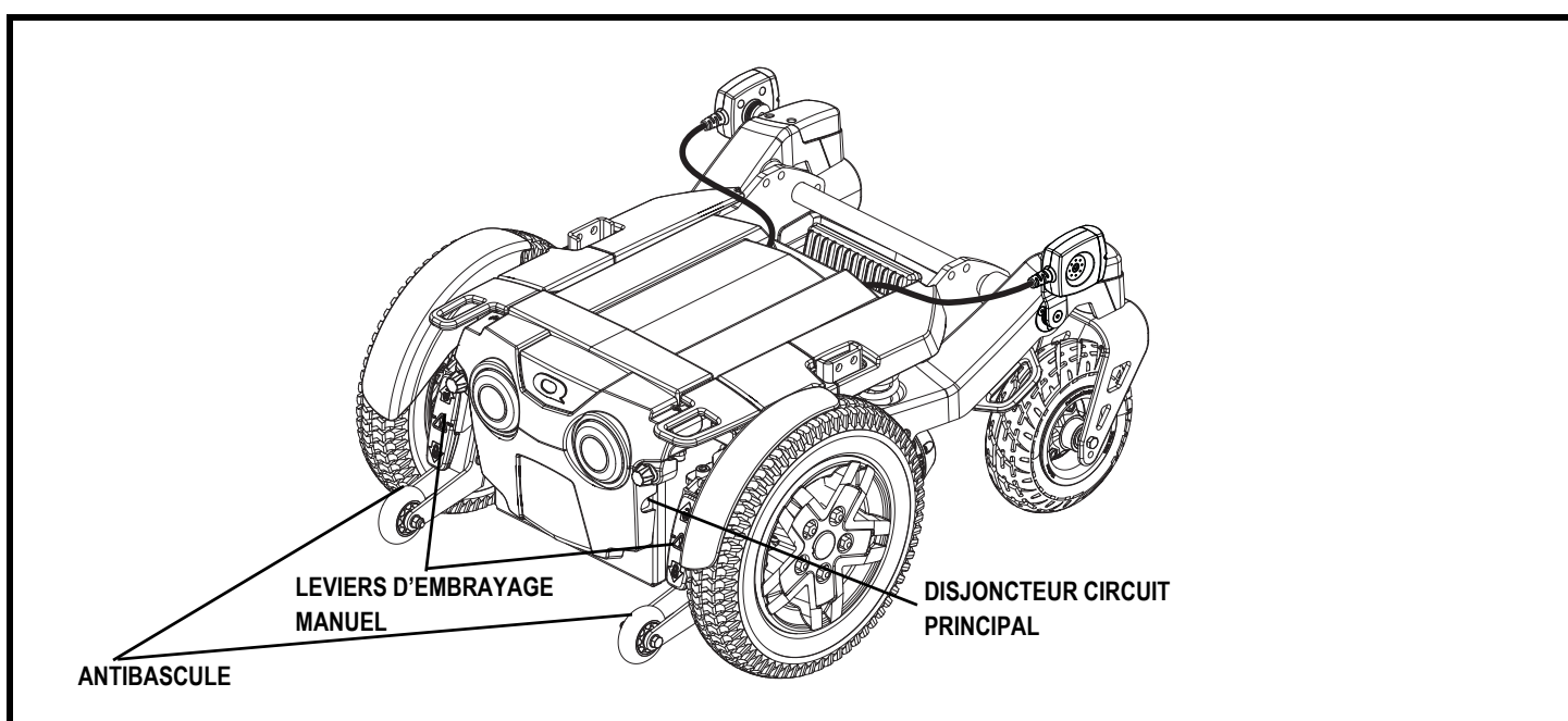
Figure 6. Base motorisée du Lightning
